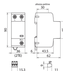
Dimensioni DSH B TT 2P 255 FM
