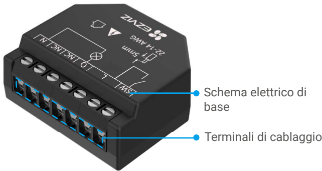
Vista anteriore
