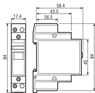
Tipo 20.23 Morsetti a vite
