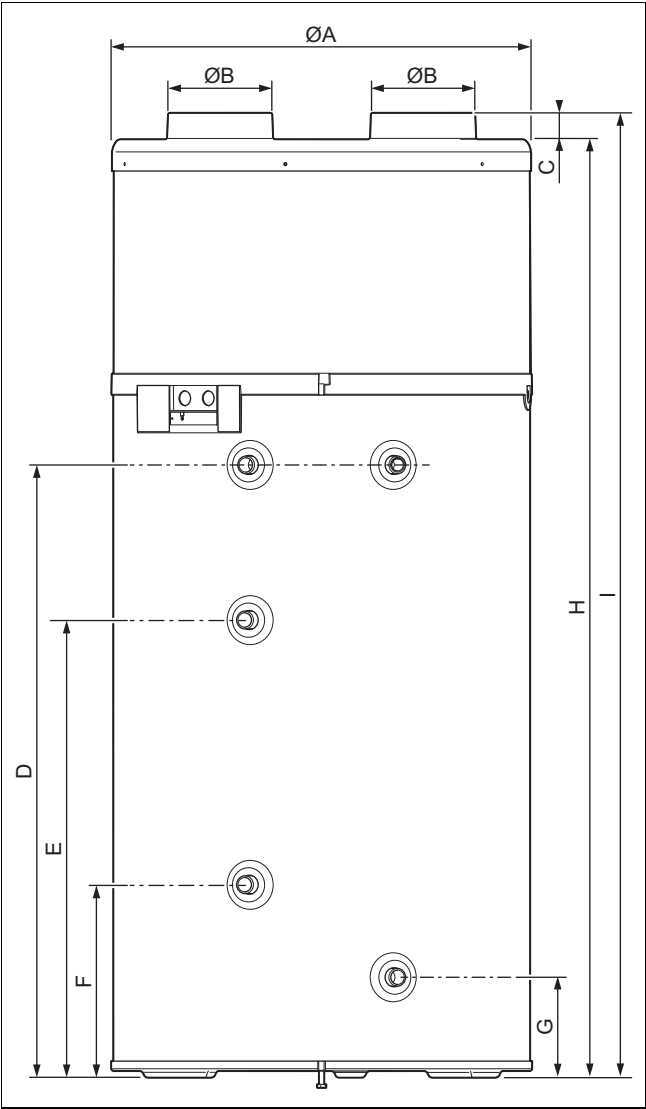
Dimensioni apparecchio e misure di raccordo con 200 e 270 l (→ Pagina 11)
